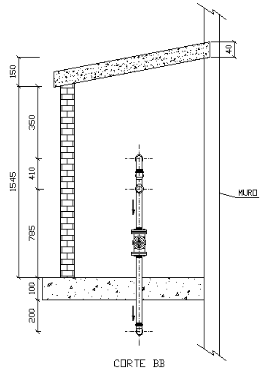
CORTE BB
