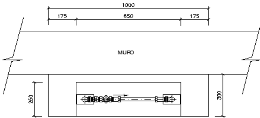
CORTE BB
