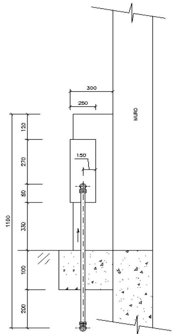
CORTE AA
