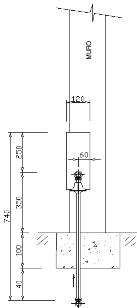
CORTE AA
